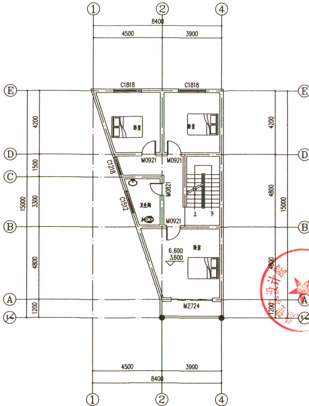
二~三层平面图 1:100
