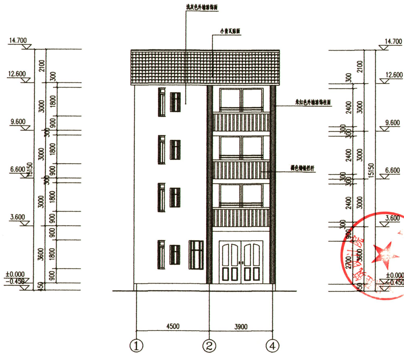
正立面 1:100
