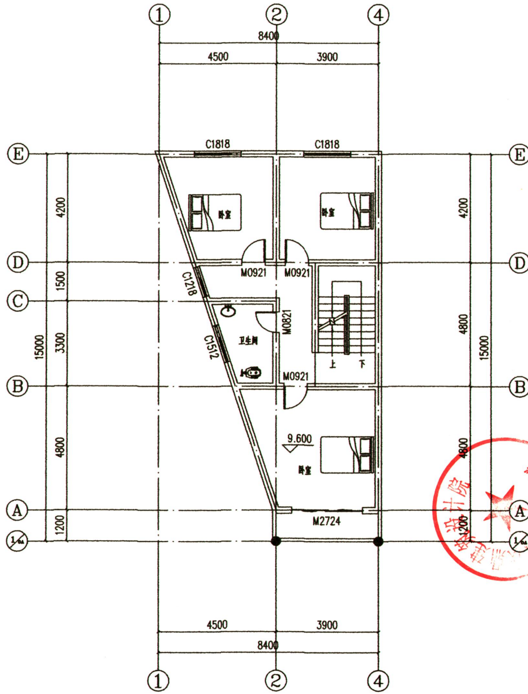
四层平面图 1:100 建筑面积 94.28m 2
