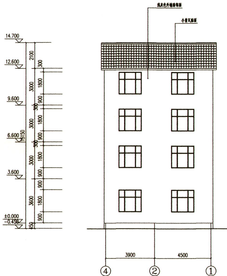
背立面 1:100
